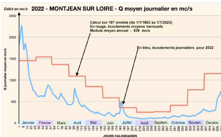
Graphe N 3 Débit (écoulement journalier) de la Loire à Montjean sur Loire (49)
